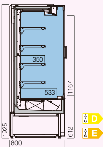
MUXV80 3M1 (-1...+5 °C) 3M2 (-1...+7 °C) dim. 625 | 937 | 1250 1562 | 1875
