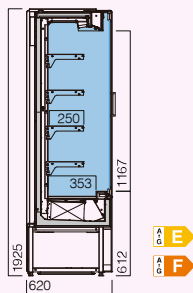
MUXV62 3M1 (-1...+5 °C) 3M2 (-1...+7 °C) dim. 625 | 937 | 1250 1562 | 1875
