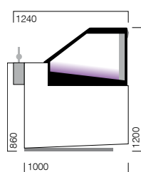
VDS GL - VD vitruina gelados ice cream display case 4L1 (-18... -15 °C) 4G3 (-18... -10 °C) DIM. 1105 | 1605 (d) | 2100 (d)
